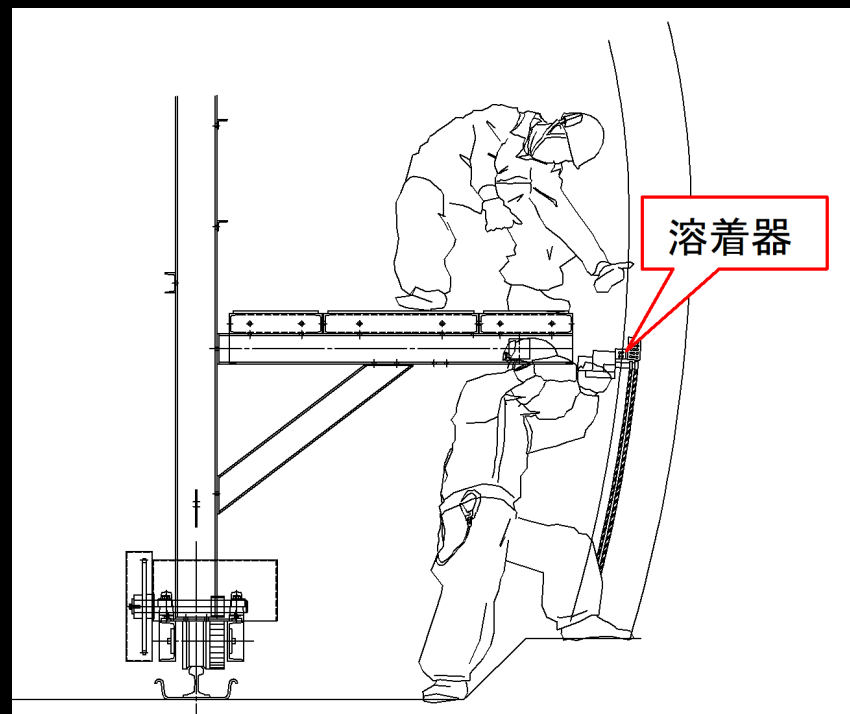
底部施工時
